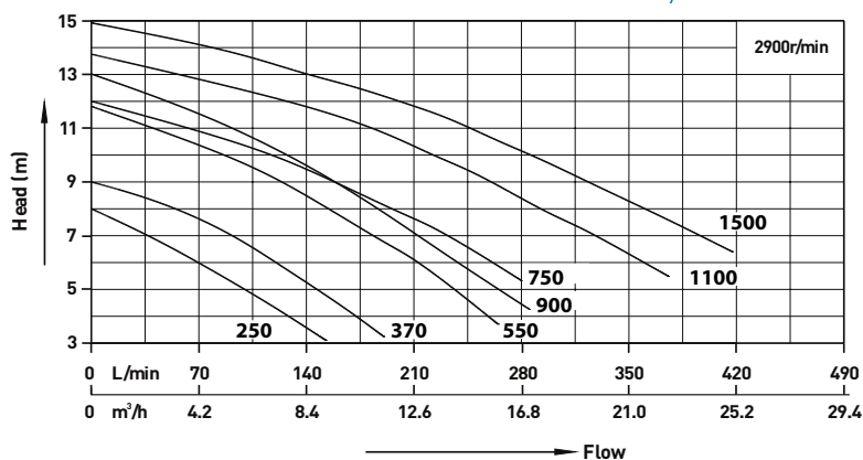
výkonnostní křivka
